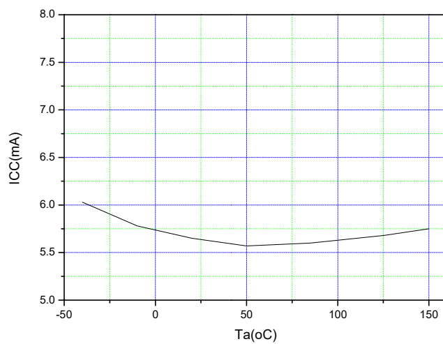
静态电流 vs. Ta
