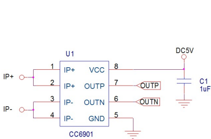
典型双端输出应用
