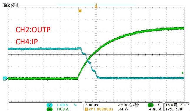
Vo vs. IP (正向电流响应)
